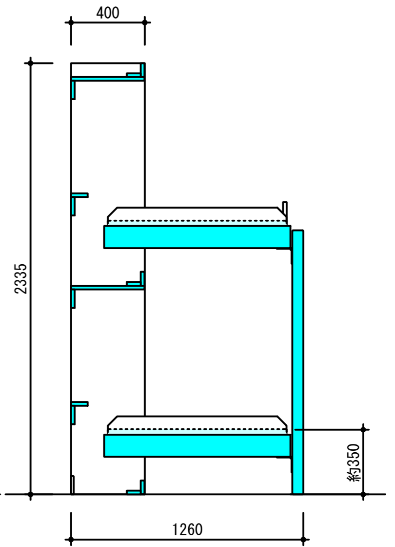
断面图
